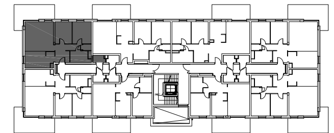
kondygnacja 1 - parter
